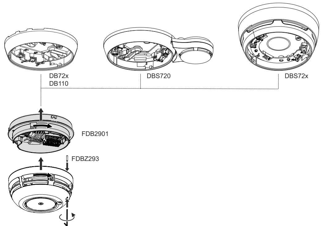
Fig. 2: Sockeladapter FDB2901 montieren
