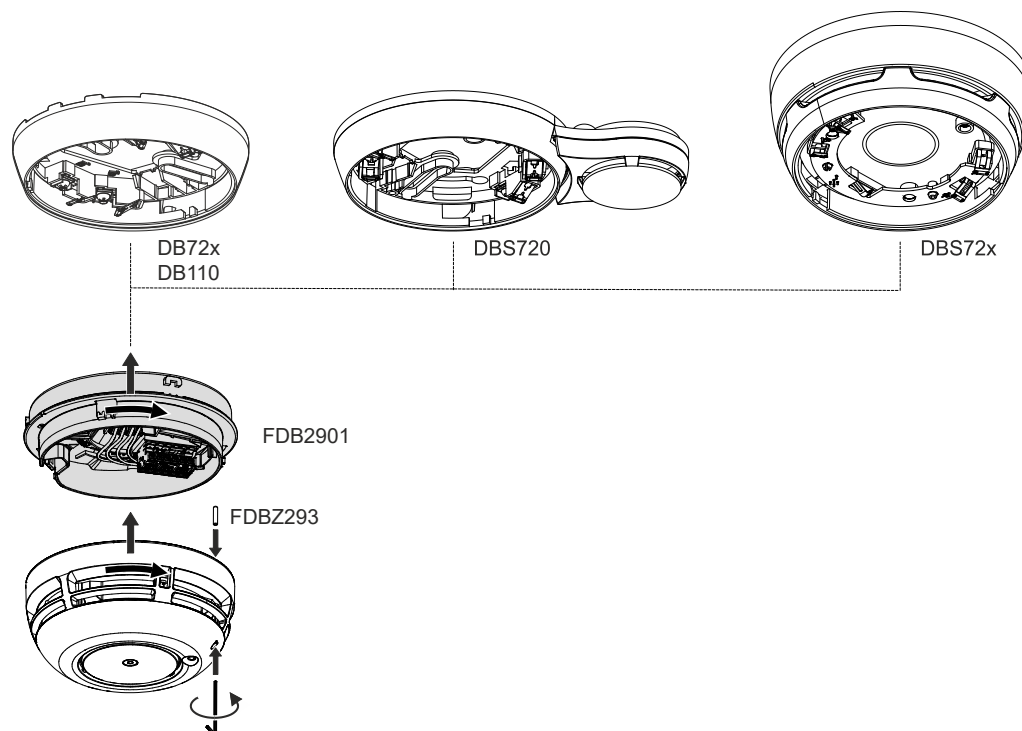
Fig. 3: Montage de l'adaptateur d'embase FDB2901
